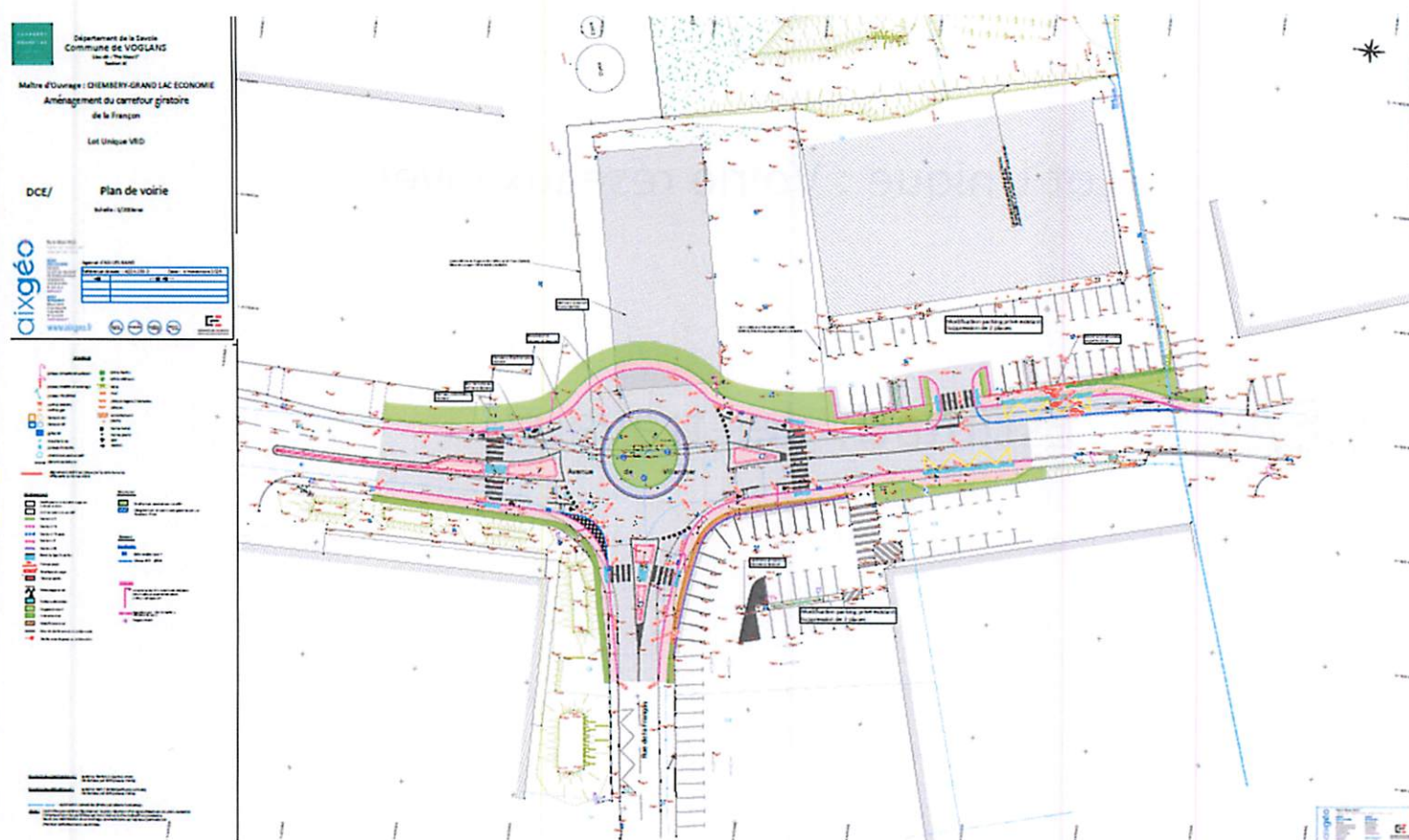
Figure 5 : Extrait plan masse projet
